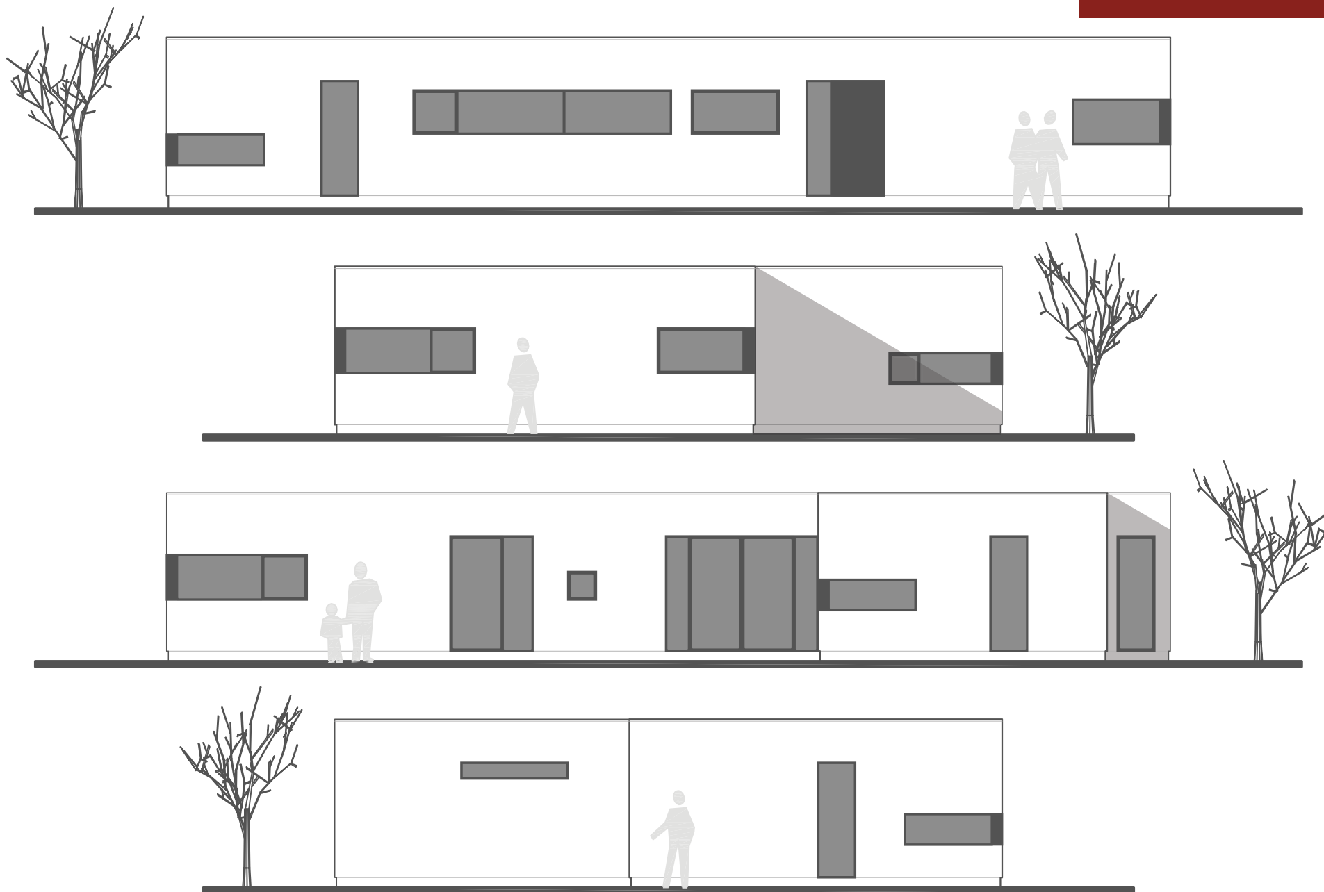
CasaBo type csb5 • retvendt model • 1:100
