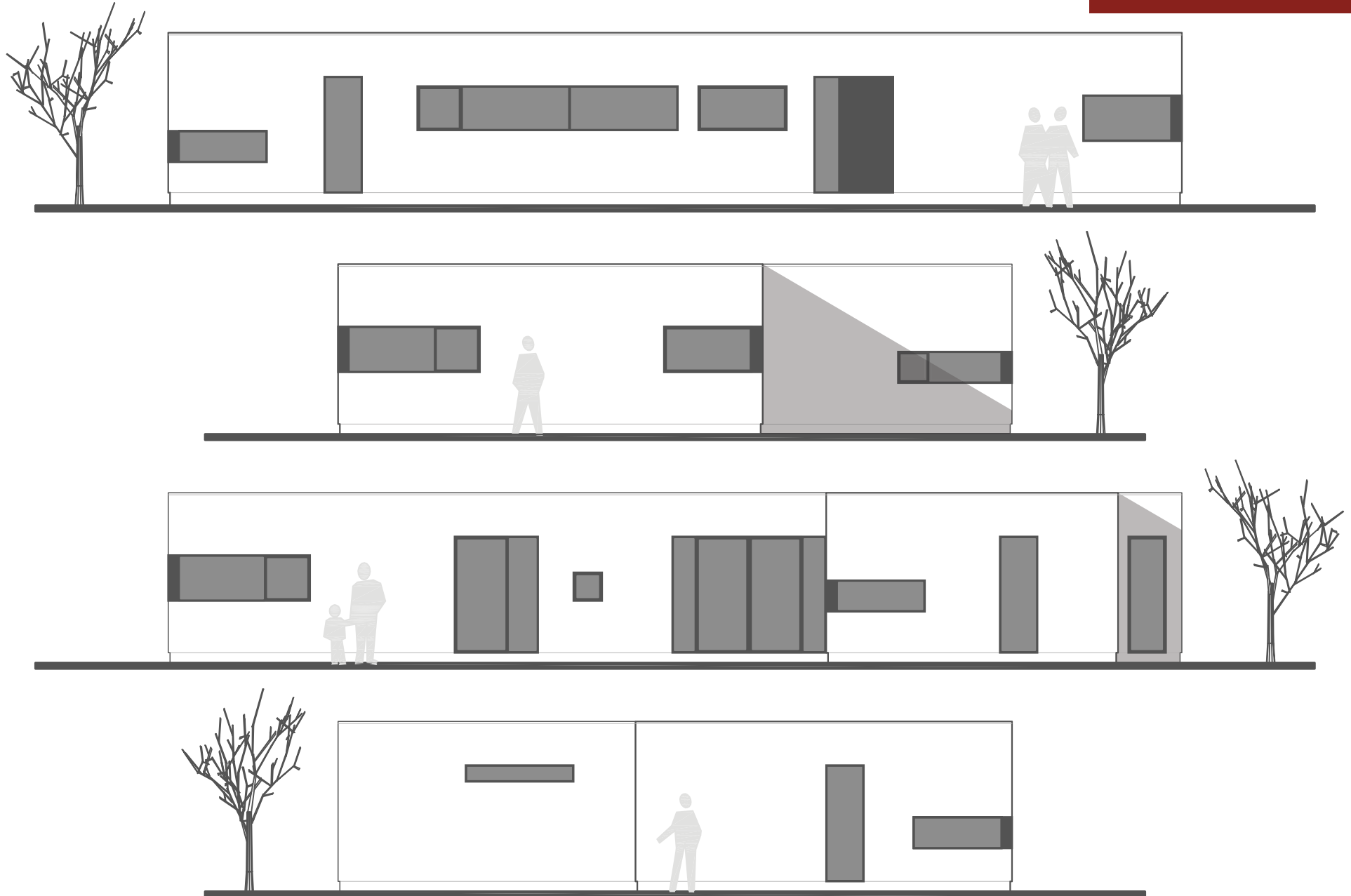
CasaBo type csb5 • retvendt model • 1:100
